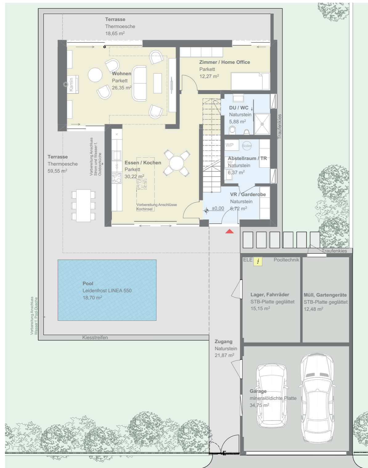
Erdgeschoss Wohnfläche 88 m 2 Terrassen 78 m 2 Nebengebäude 62 m 2
