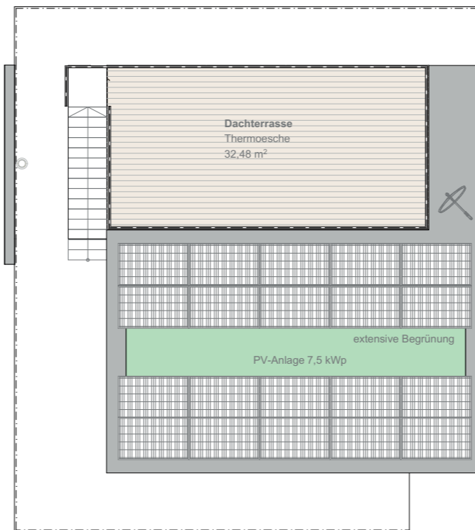
Dachgeschoss Terrasse 32 m 2
